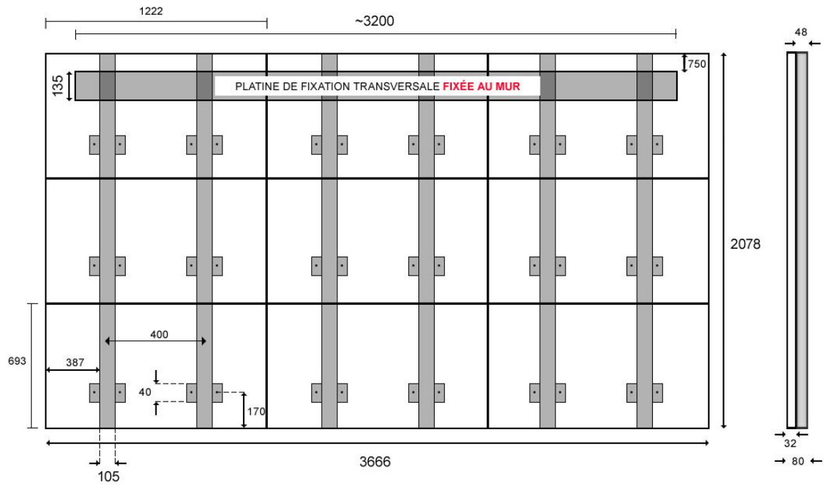
Cotes d'un mur 3x3 horizontal
