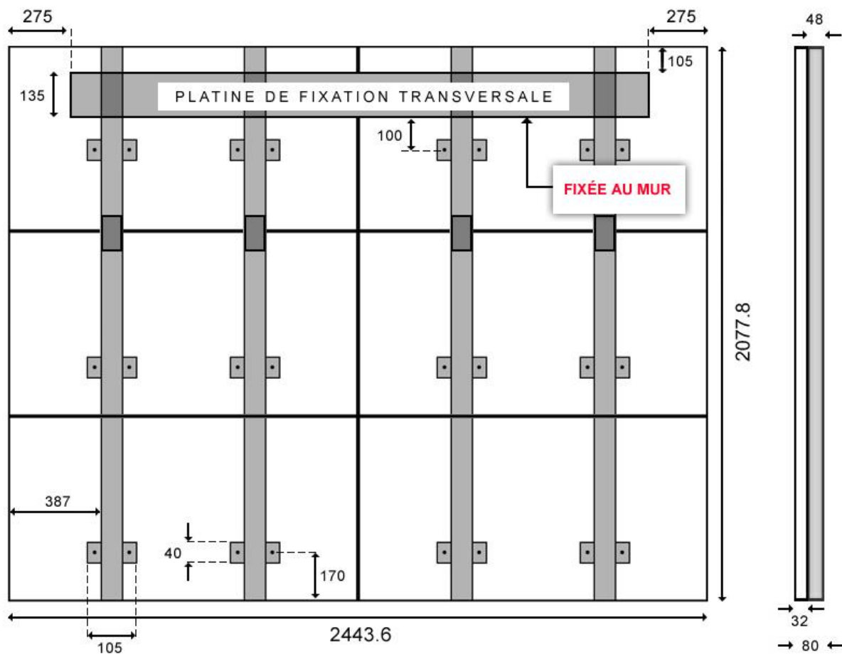
Cotes d'un mur 3x2 horizontal
