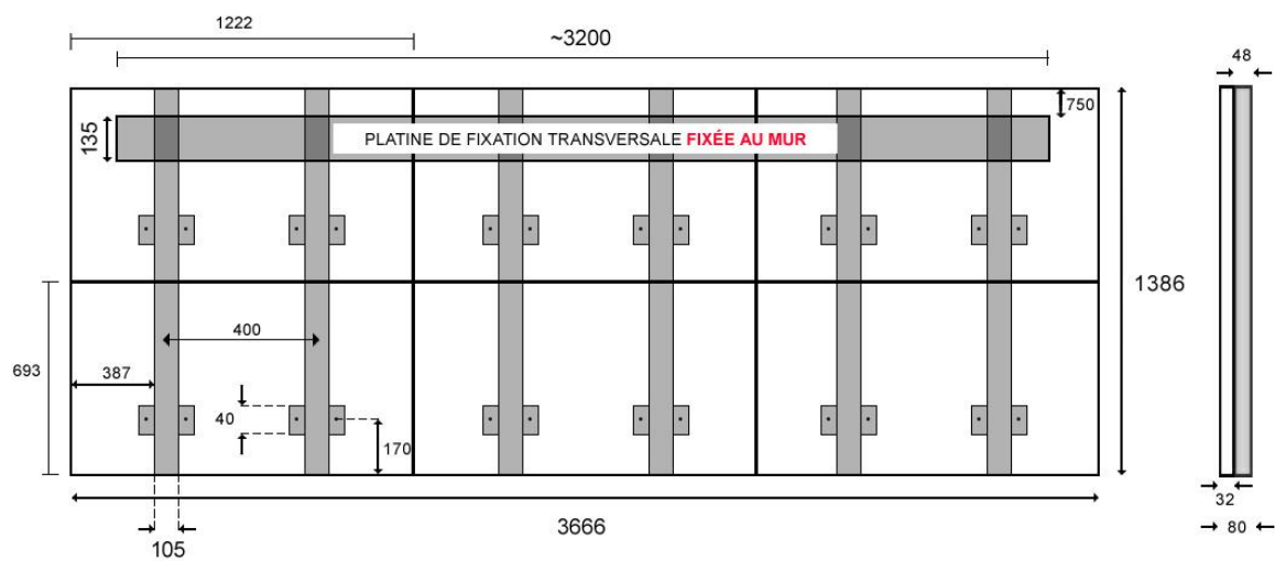
Cotes d'un mur 3x2 horizontal
